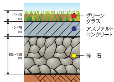
新設時推奨断面 (アスコン)
