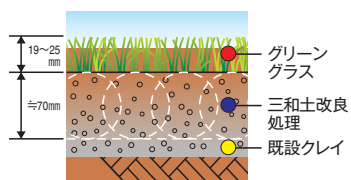
改修時推奨断面
