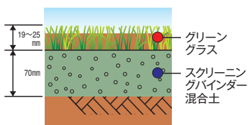
新設時推奨断面 (SB工法)
